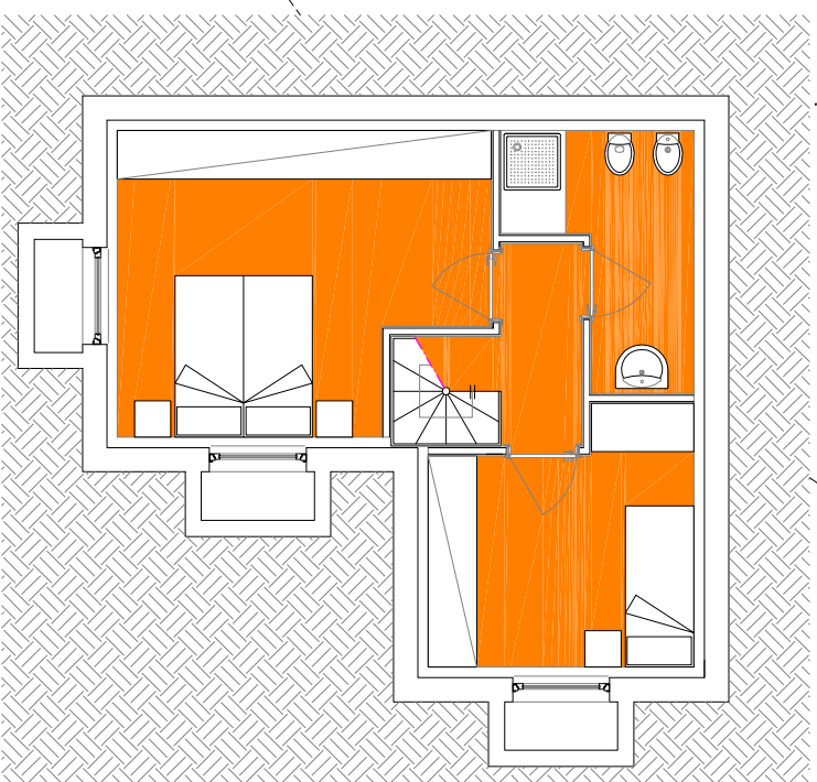
Pianta piano interrato Ipotesi B
